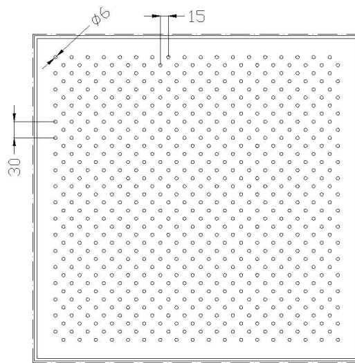
PLACA TIPO 2A \phi 6mm PASO 1: 15mm, PASO 2: 30mm APERTURA 4,9%
